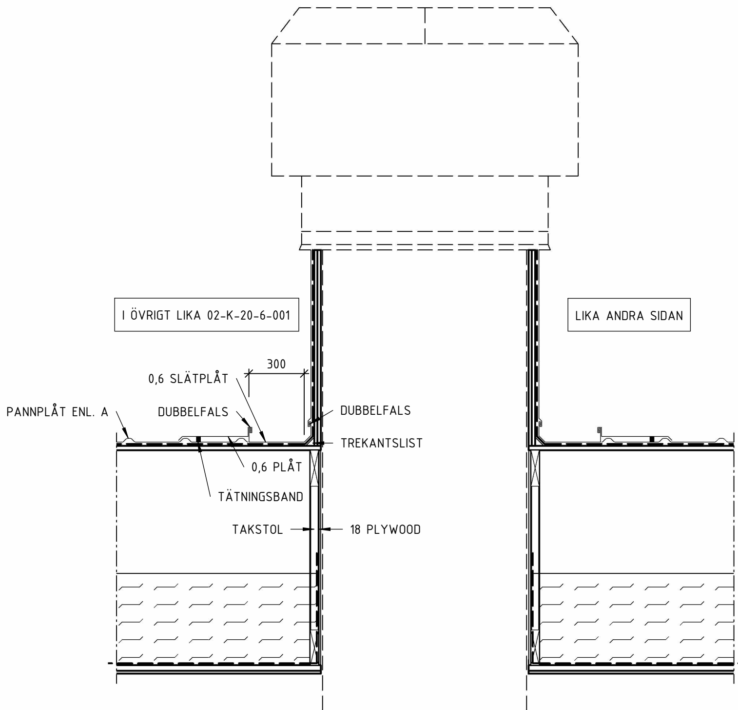
11 1 : 20 PRINCIPDETALJ TAKHUV
