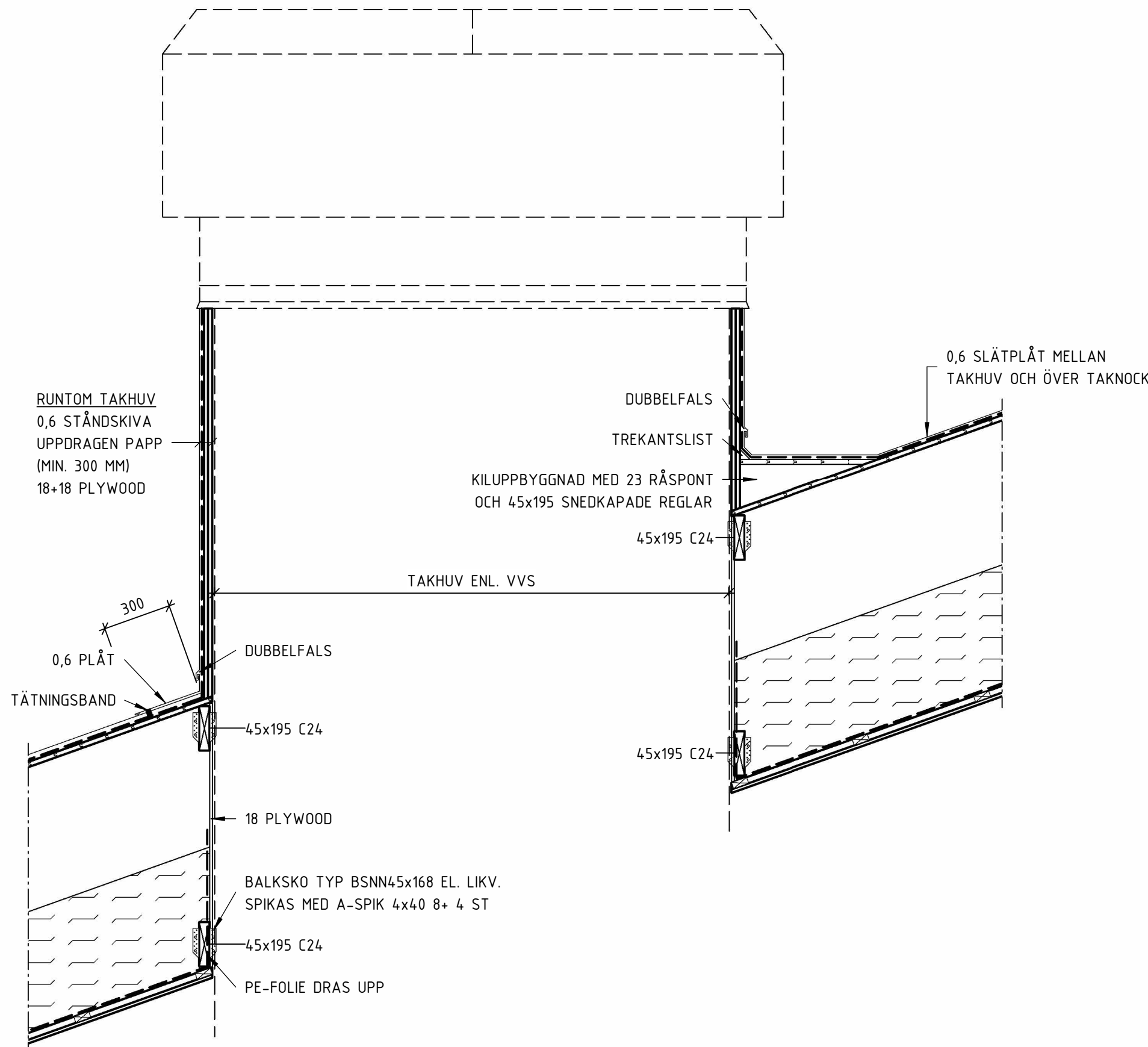
10 1 : 20 PRINCIPDETALJ TAKHUV
